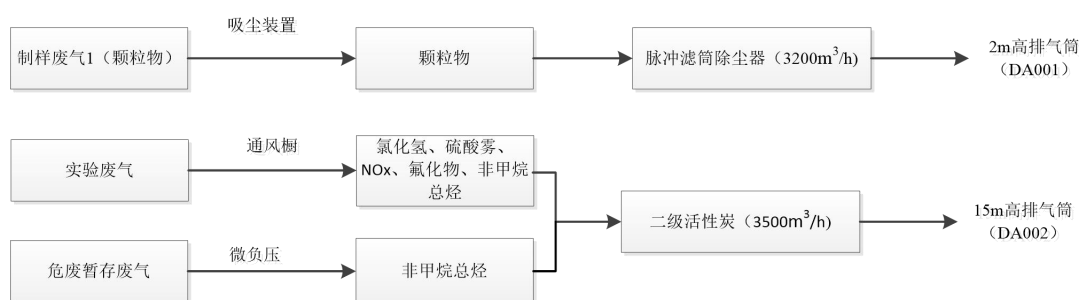
图 4-1 废气收集、处理方式示意图
