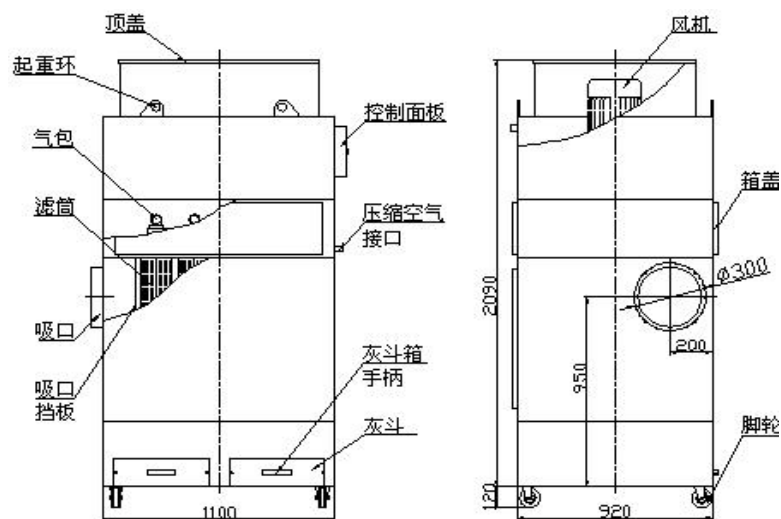
图 4-2: 除尘器工作原理图
