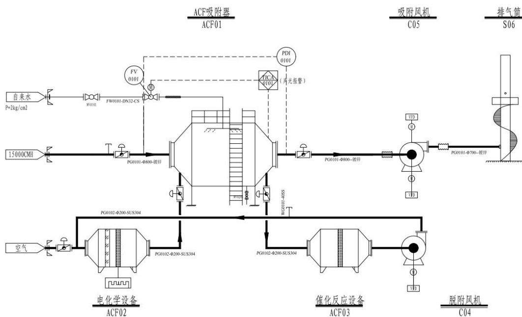
图 4.2-3 甲类仓库及危废库废气处理流程示意图
