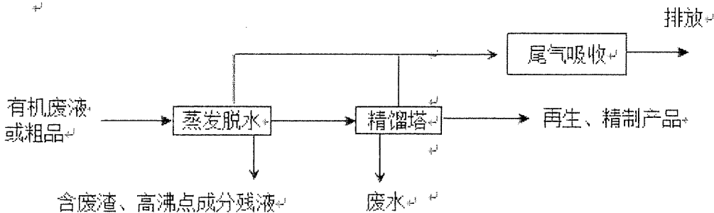
图 3-1 化学品再生、精制的工艺原理图
