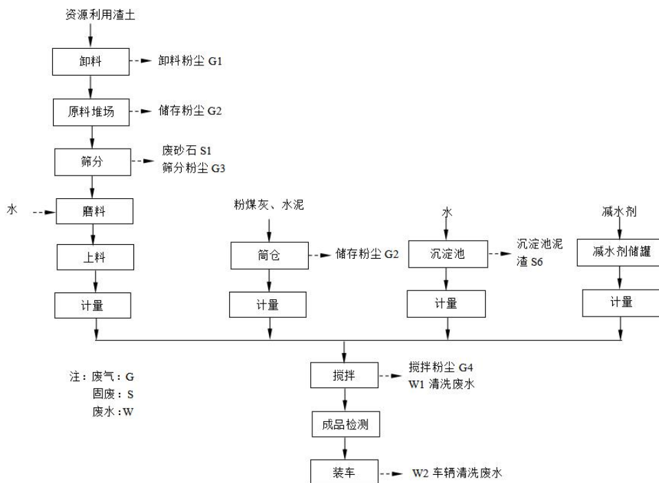
图 2-4 流态固化土生产工艺流程图
