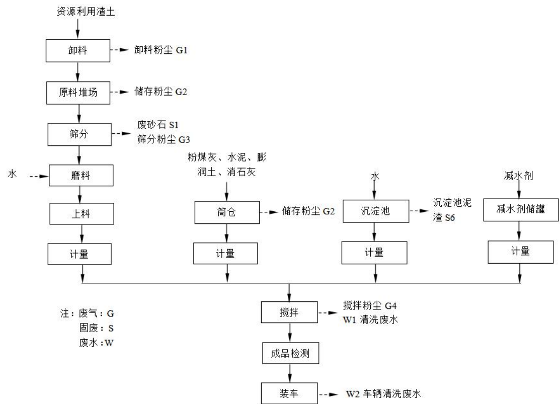
图 2-3 地铁盾构同步注浆浆液生产工艺流程图
