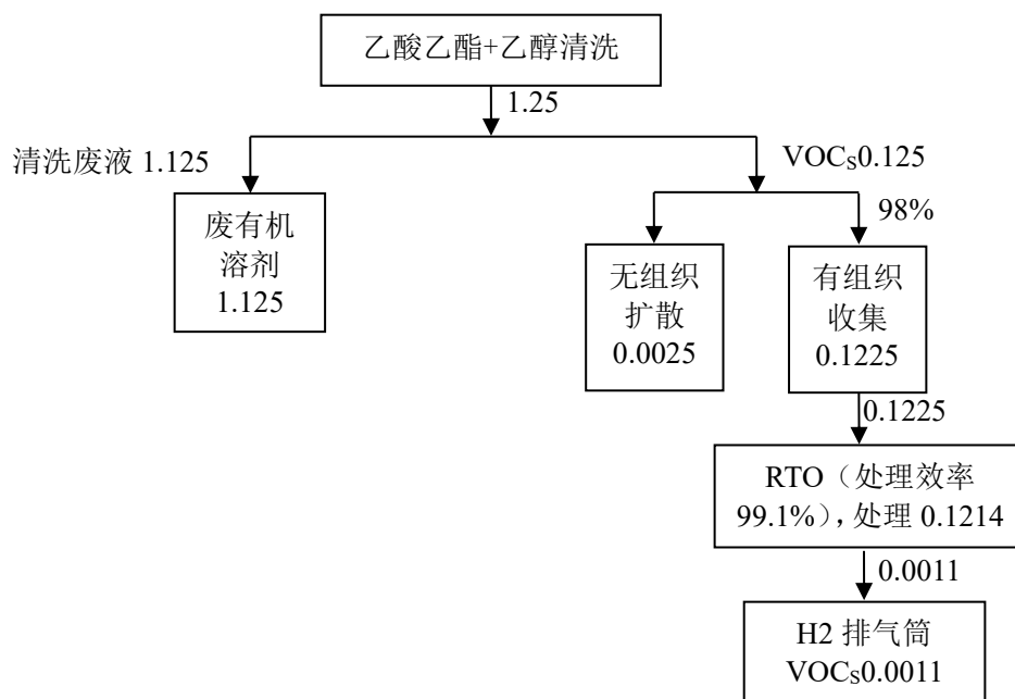
图2-2 建设项目乙酸乙酯+乙醇清洗物料衡图（t/次）
