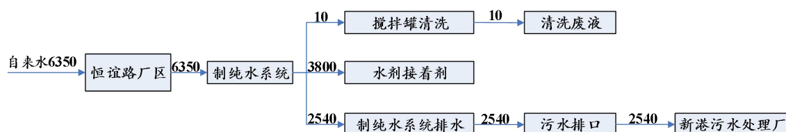
图2-4 本次扩建项目水平衡图（t/a）
