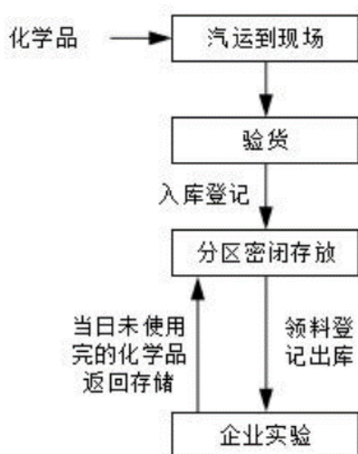
图 4.2-3 本项目危化品入库工艺流程
