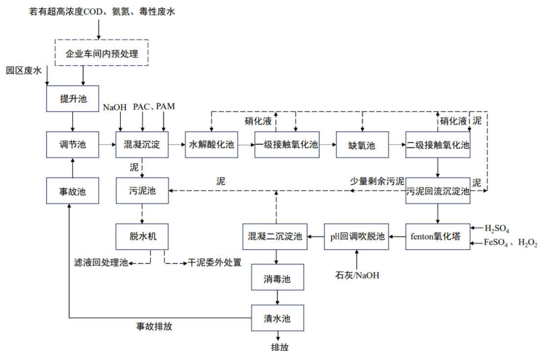
图 4.2-2 本项目废水处理工艺流程
