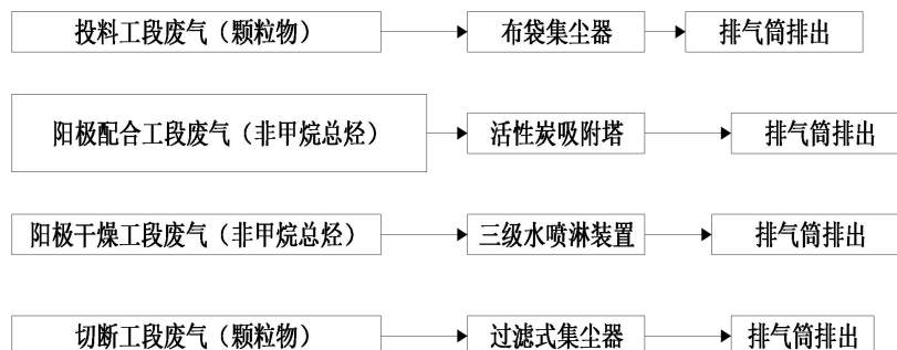
图 4-1 废气收集、治理、排放流程示意图
