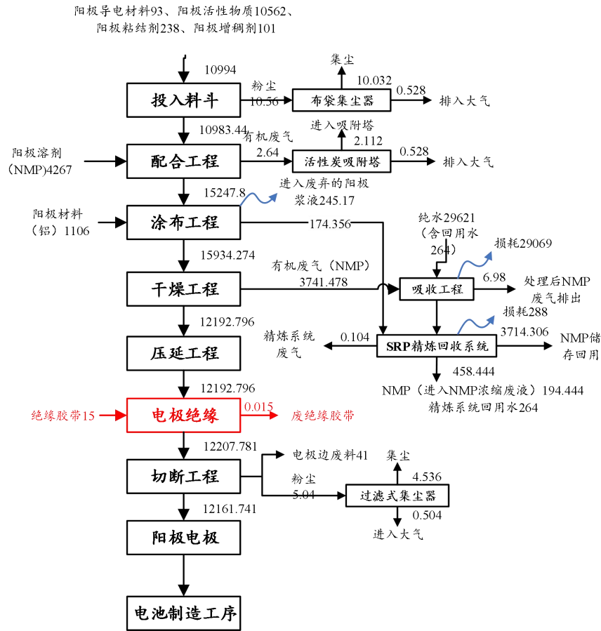
图2-3 八工厂11~12号阳电极生产过程物料平衡图 (t/a)
