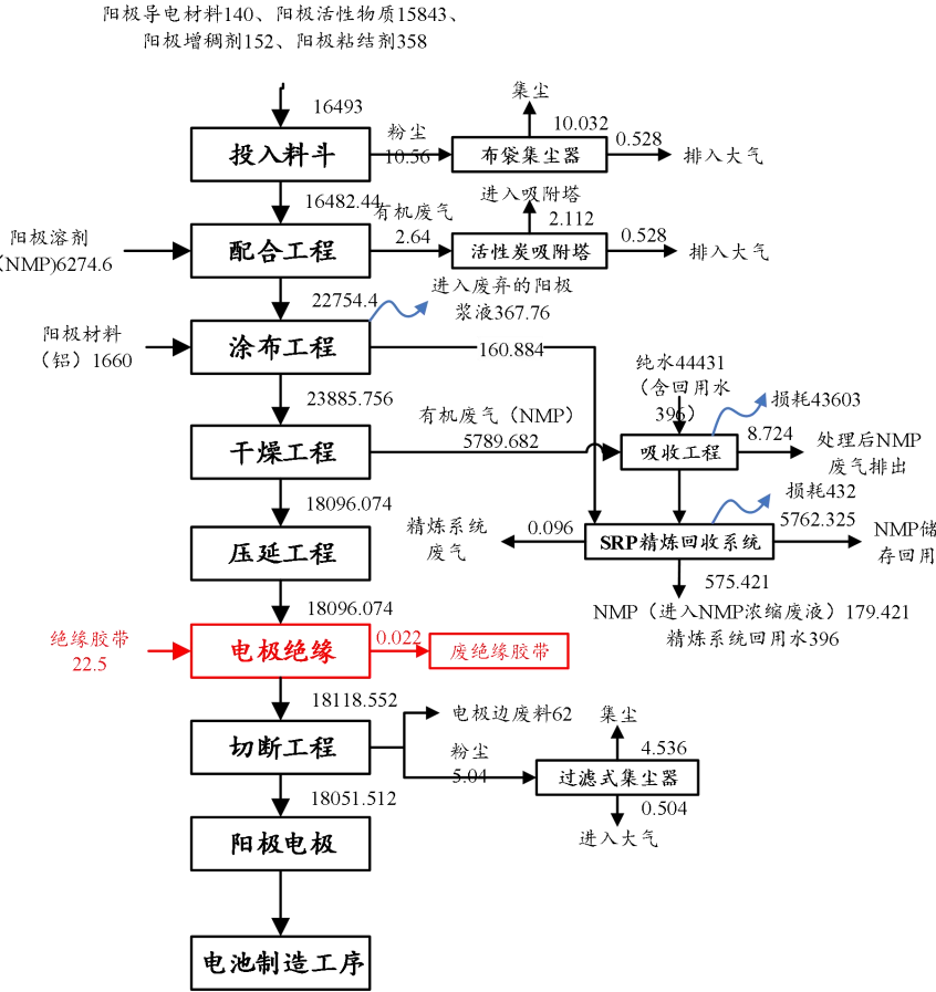
图2-1 一工厂8~10号阳电极生产过程物料平衡图 (t/a)
