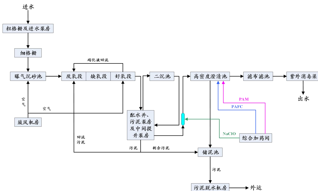
图 4-2 开发区污水处理厂污水处理工艺流程图
