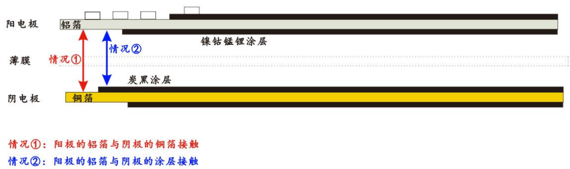
图2-6 技改前绕卷后阴极阳极接触的部分可能出现的短路现象示意图
