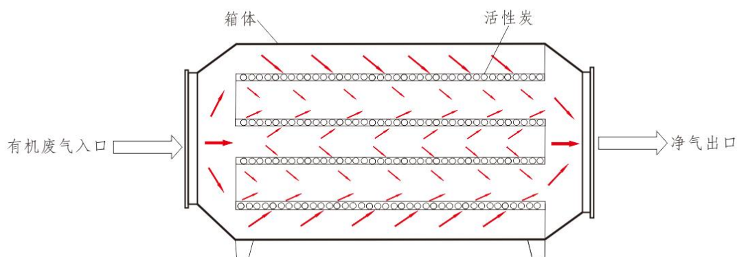
图 4-5 活性炭吸附塔结构示意图
