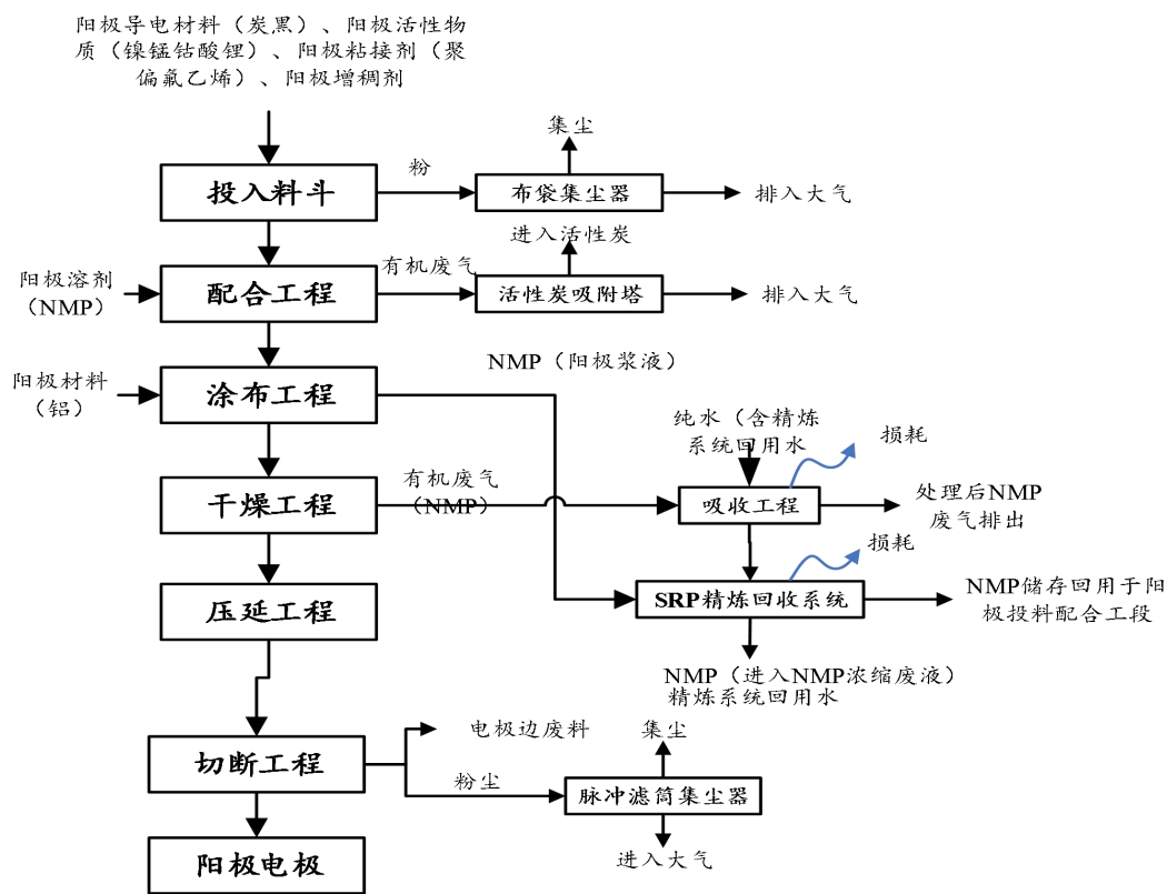
图 2-7 原阳极产线工艺流程图
