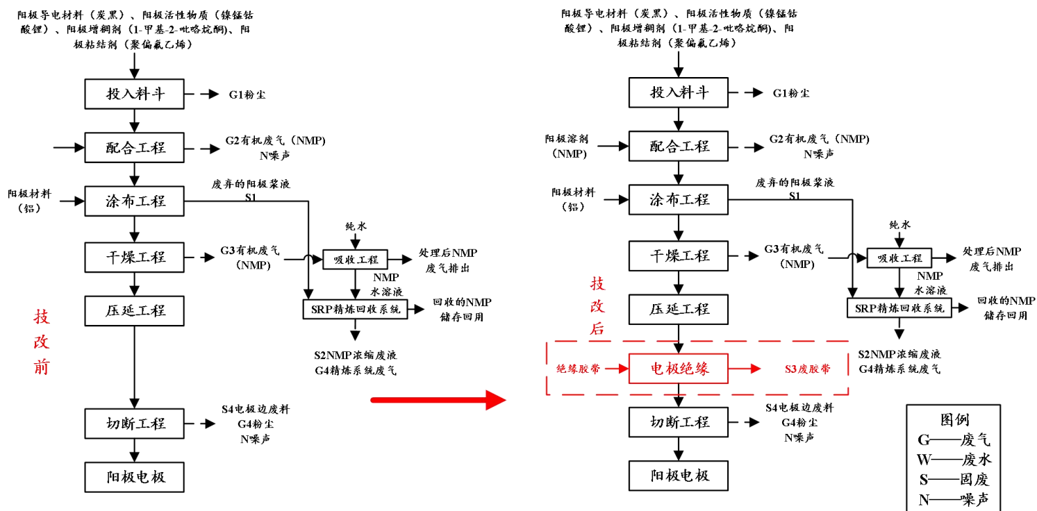
图2-5 阳电极工艺流程及产污节点示意图
