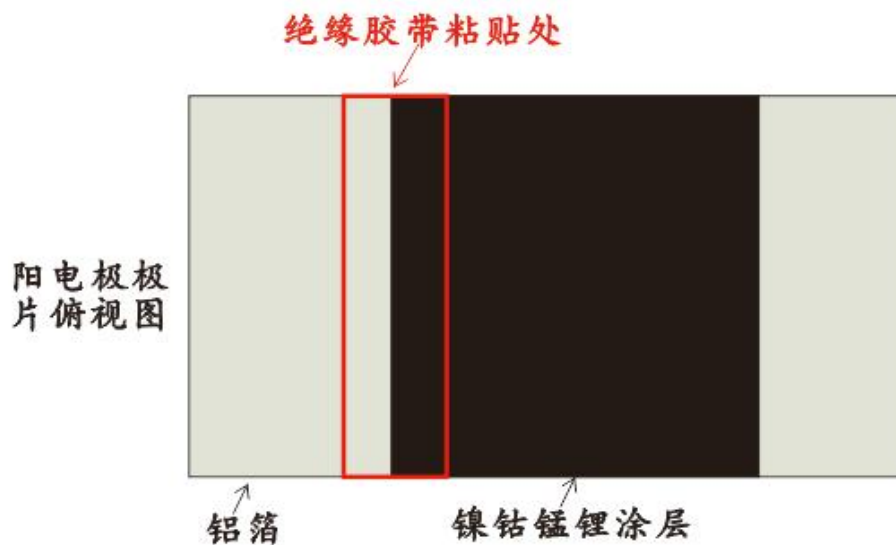
图2-7 技改后阳电极可能出现的短路的部分缠绕绝缘胶带示意图
