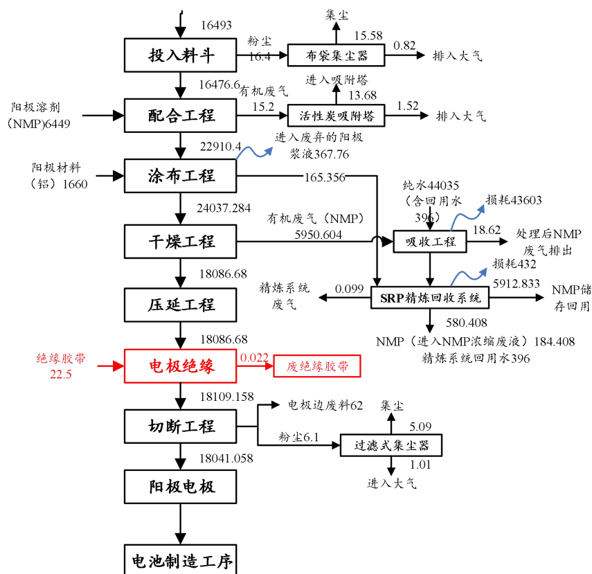
图2-2 七工厂5~7号阳电极生产过程物料平衡图 (t/a)
