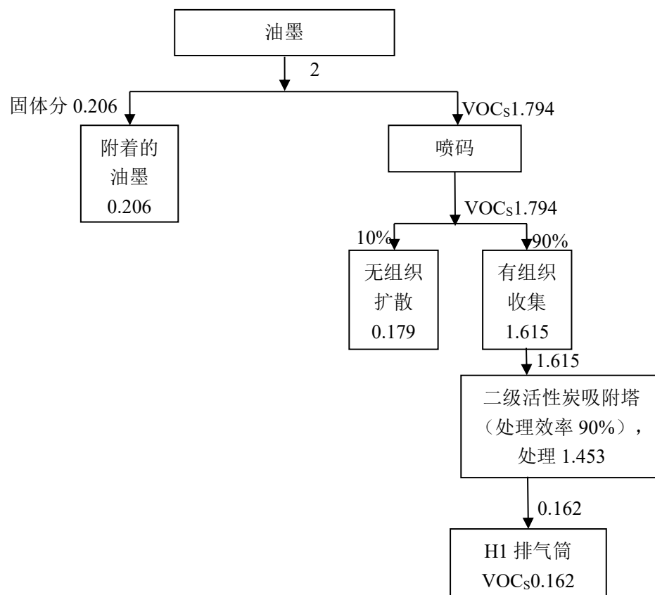
图2-1 建设项目喷码油墨平衡图 (t/a)
