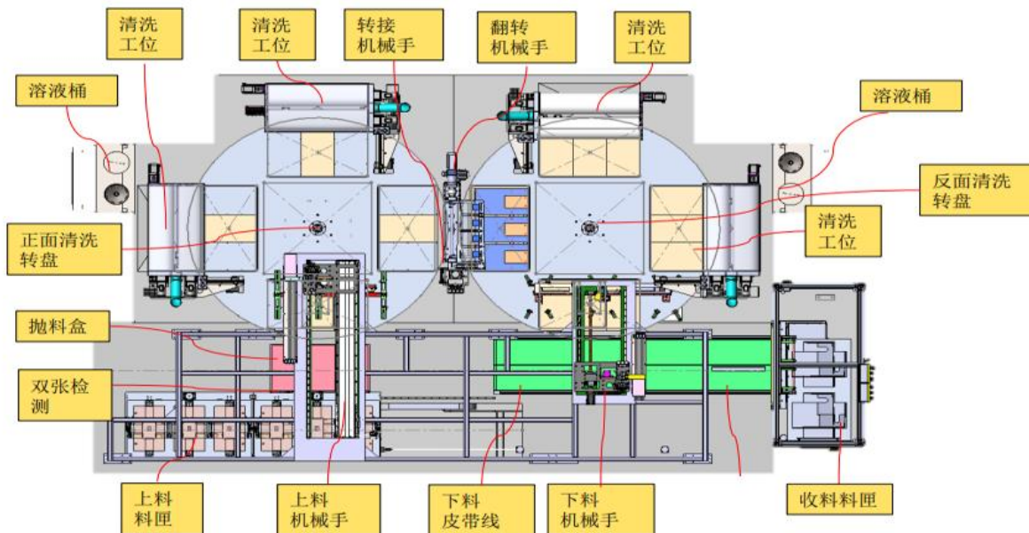
图2-6 擦胶机工作原理示意图
