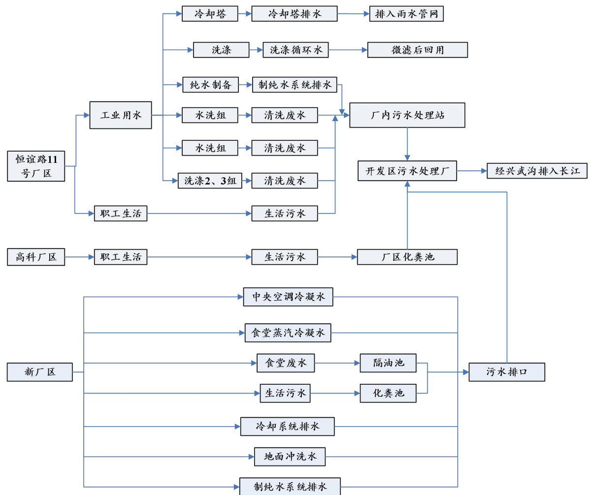
图2-11 现有项目废水产生及治理情况示意图
