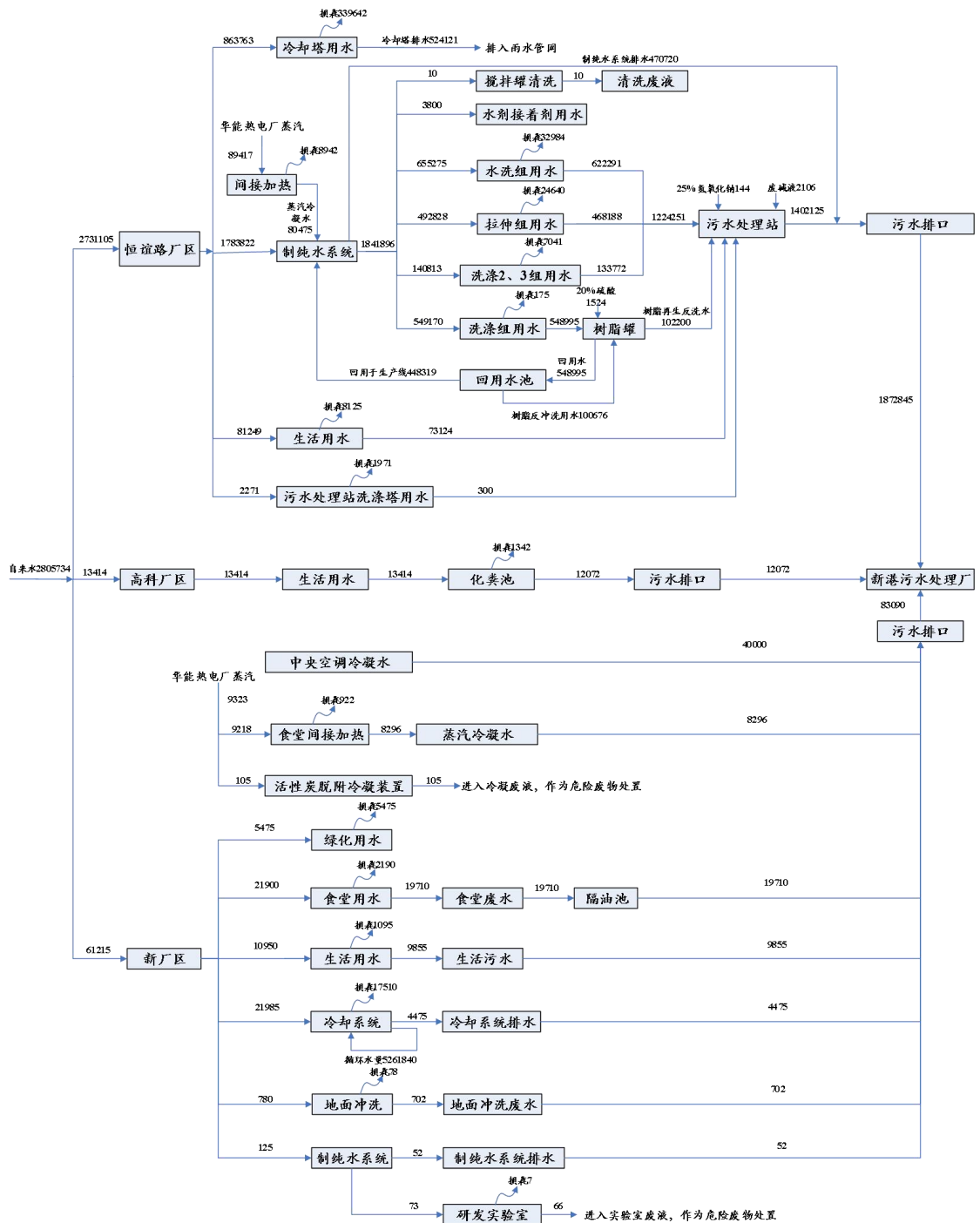
图2-4 项目建成后全厂水平衡图 (t/a)
