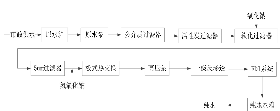
图 2-1 纯水制备工艺流程图
