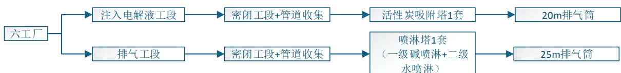
图 4-1 废气收集、治理、排放流程示意图
