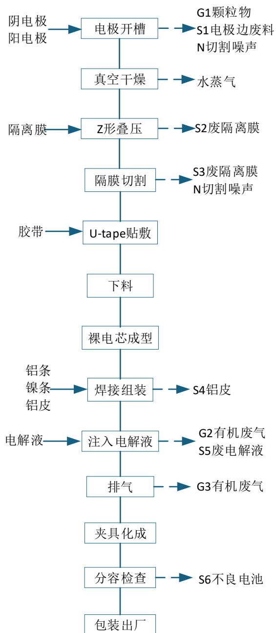
图 2-8 现有项目 ZZS1.5 POUCH 型锂离子电池工艺流程及产污环节图
