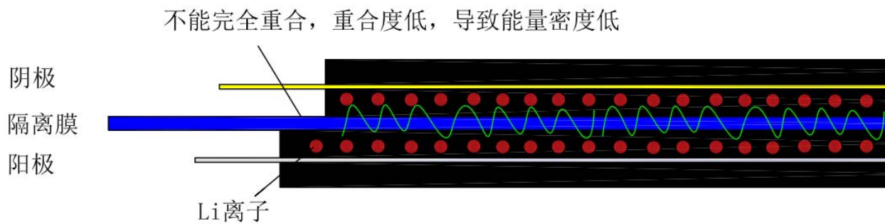
图2-6 技改前“堆叠”工段示意图（电极与电极之间形状差异大）
