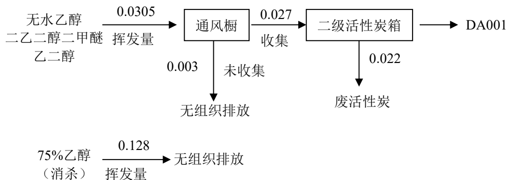
图 4-1 全厂 TVOC 平衡图 (t/a)
