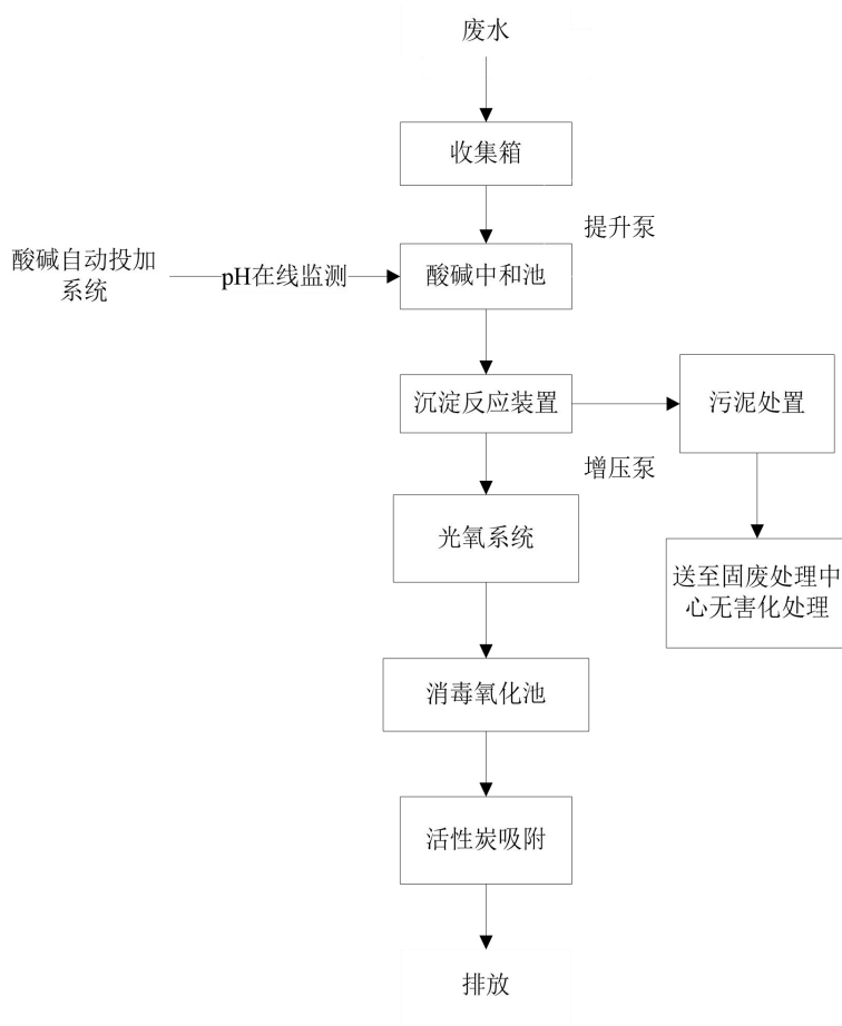
图 4-3 厂区废水预处理工艺流程图
