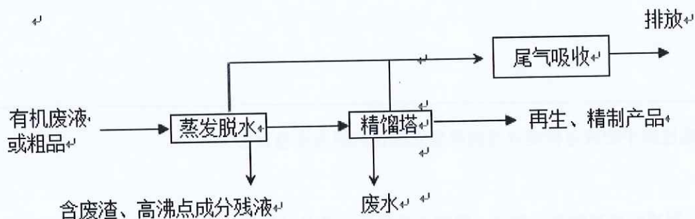
图 3-1 化学品再生、精制的工艺原理图
