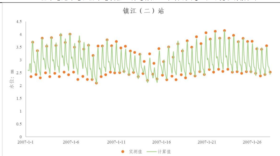
图 5.2.2-5 镇江（二）站计算值与实测值对比图
