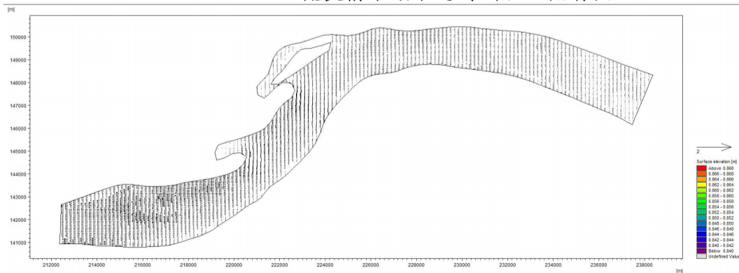
5.2.2-10 (a) 疏浚前小潮落急时刻长江流场图
