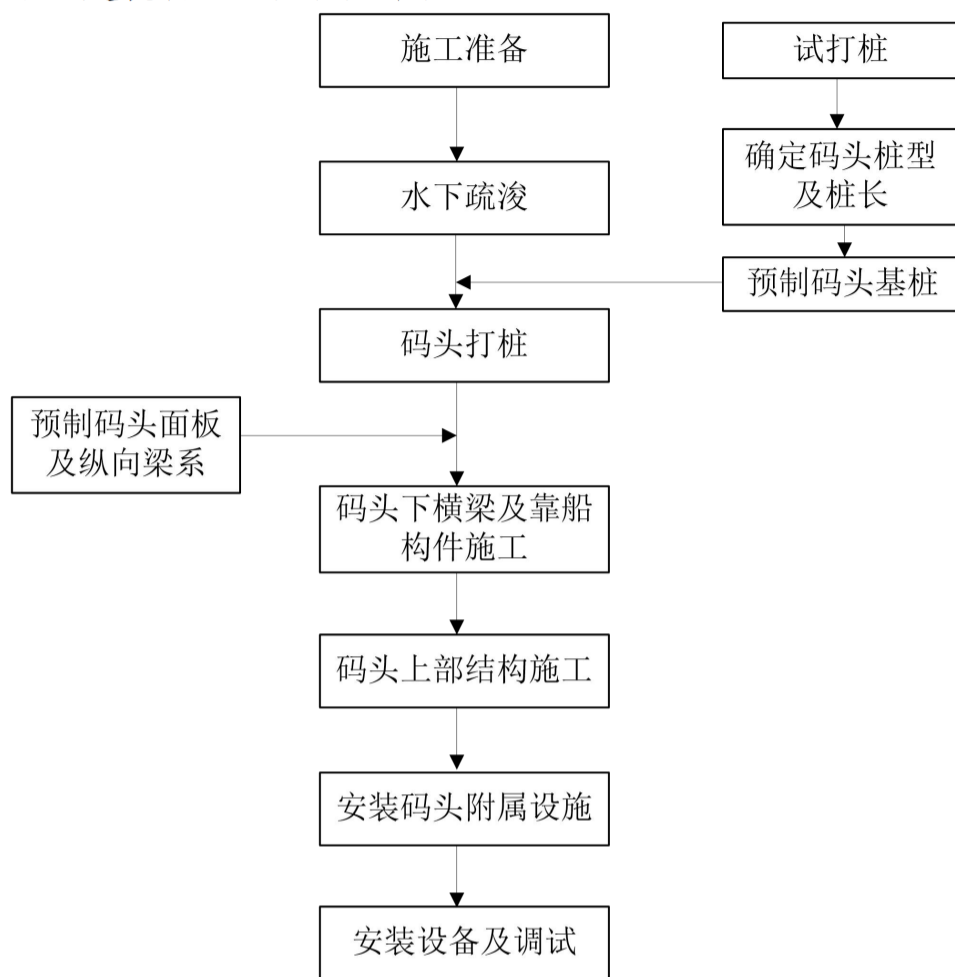
图 3.2.8-2 水工建筑物施工流程图
