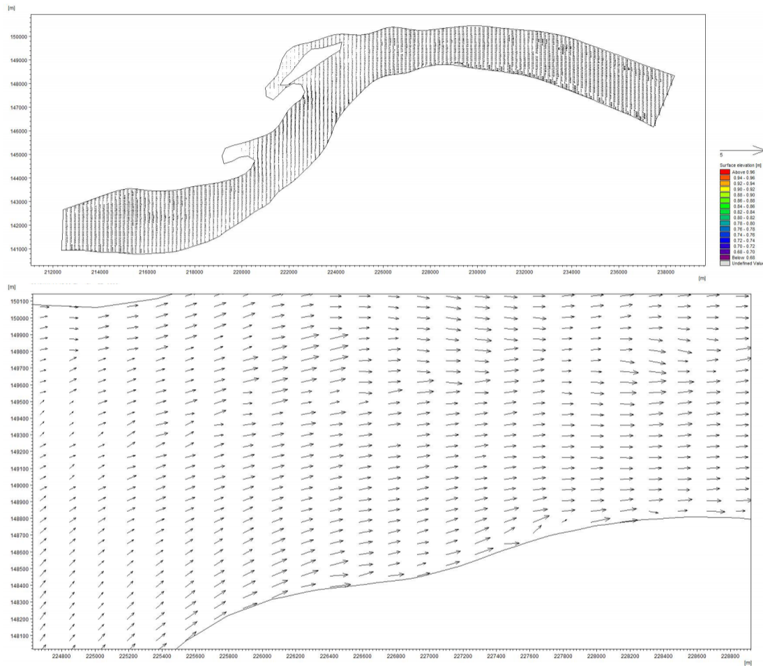
5.2.2-10 (a) 疏浚前小潮落急时刻长江流场图
