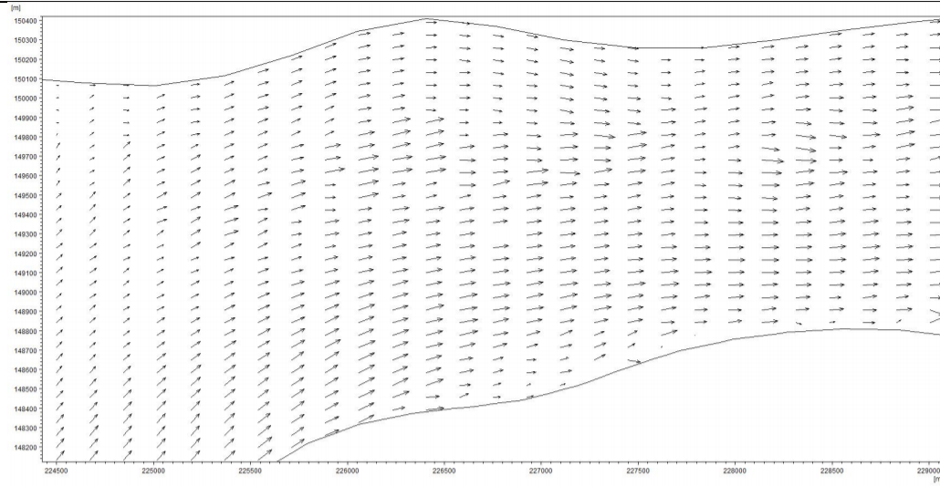
5.2.2-12 (a) 疏浚后小潮落急时刻长江流场图
