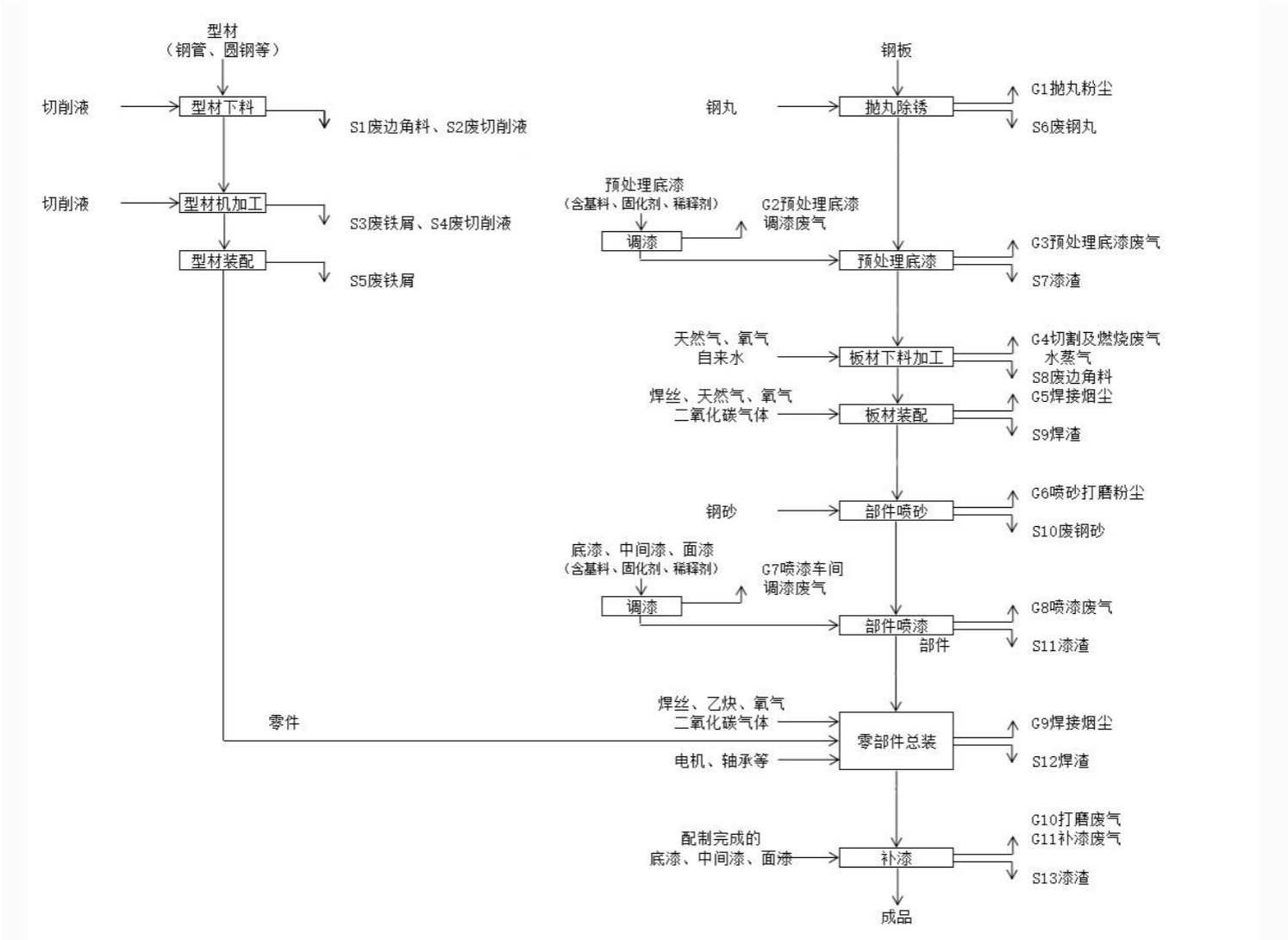
图 3.1.3-2 港机产品生产工艺流程图
