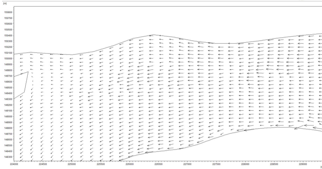
5.2.2-11 (b) 疏浚前大潮涨急时刻长江流场图
