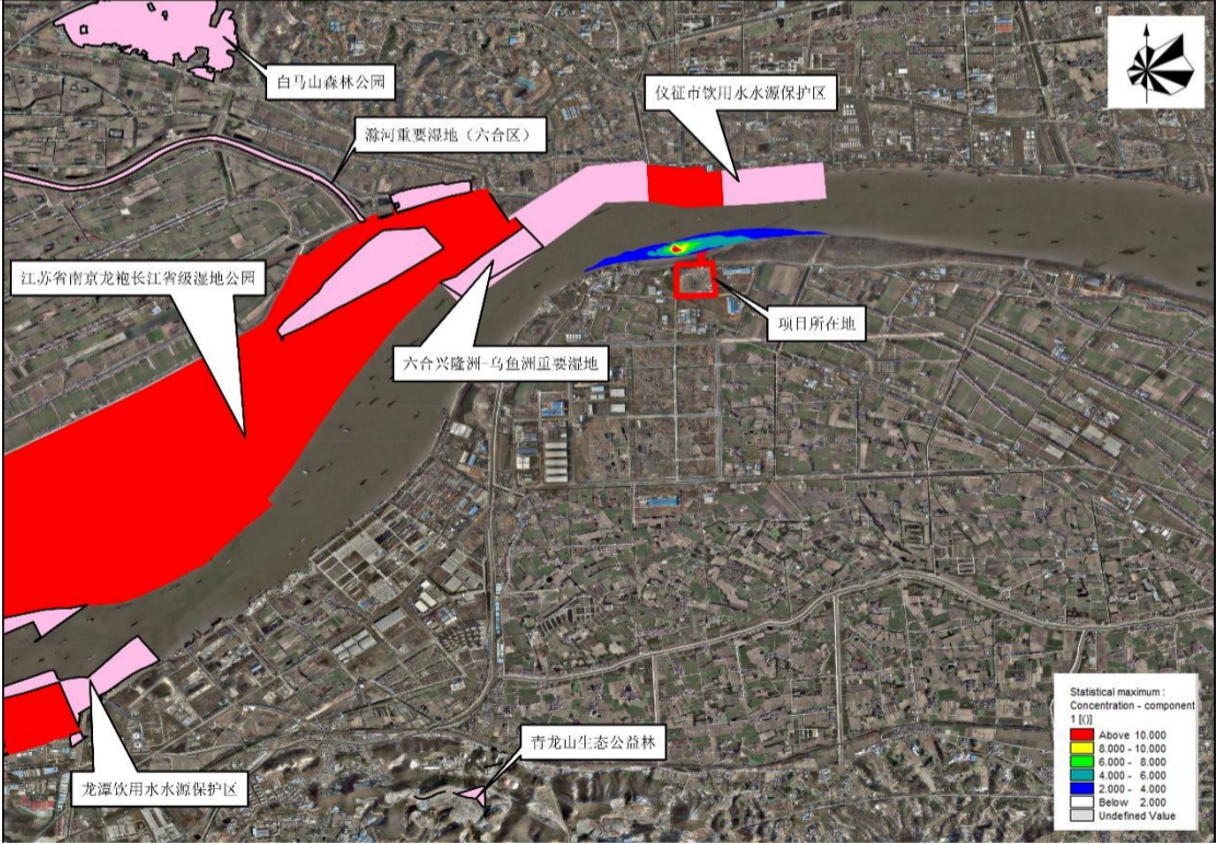
图 5.1.2-3 典型枯水期大潮悬浮物最大浓度增量分布包络图
