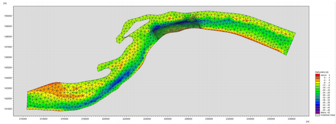
图 5.2.2-7 计算区域概化地形及网格图
