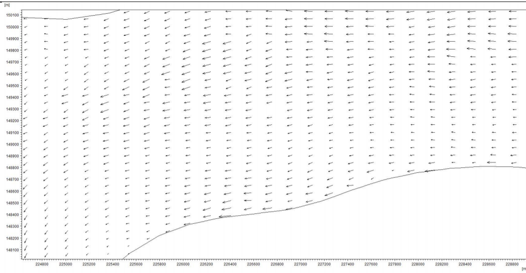
5.2.2-10 (b) 疏浚前小潮涨急时刻长江流场图
