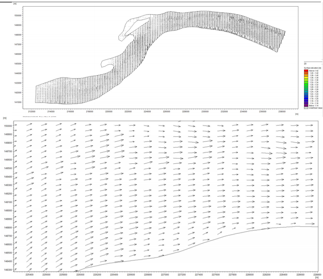
5.2.2-13 (a) 疏浚后大潮落急时刻长江流场图
