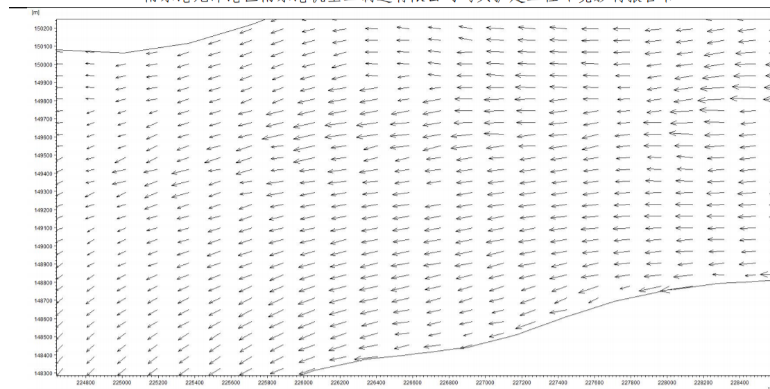
5.2.2-13 (b) 疏浚后大潮涨急时刻长江流场图
