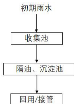
图 6.2.2-2 初期雨水处理工艺流程
