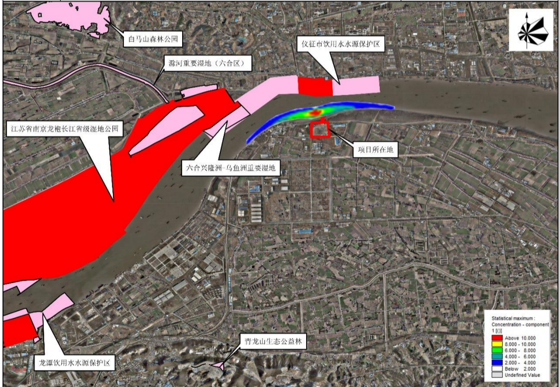
图 5.1.2-2 典型枯水期小潮悬浮物最大浓度增量分布包络图
