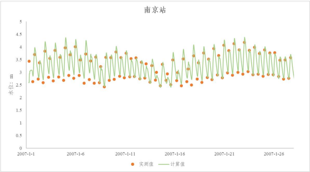
图 5.2.2-4 南京站计算值与实测值对比图
