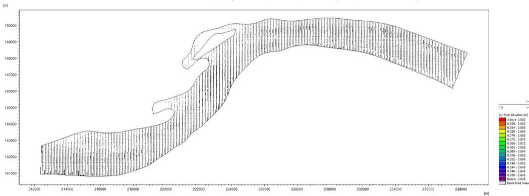
5.2.2-12 (a) 疏浚后小潮落急时刻长江流场图
